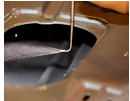
Hohlraumkonservierung Porsche
